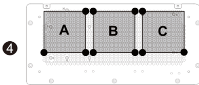
4. Схема розміщення та закріплення трьох 90 мм вентиляторів (A,B,C) на нижній панелі.
