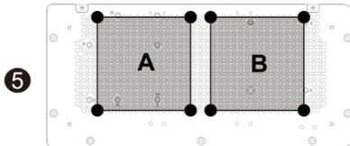
5. Схема розміщення та закріплення двох 120мм вентиляторів (A,B) на нижній панелі.
